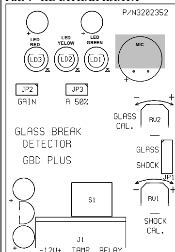
Рис. 4 - ПЕЧАТНАЯ ПЛАТА
