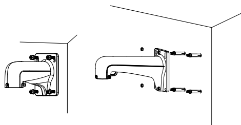
Рисунок 3-4 Установка кронштейна
