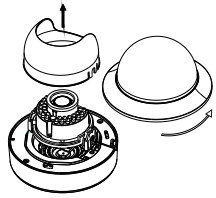
Рисунок 2-2 Снятие купола
