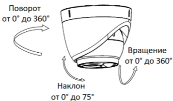
Рисунок 2-8 3-х осевая регулировка объектива
