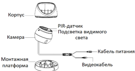
Рисунок 1-2 Камера II типа
